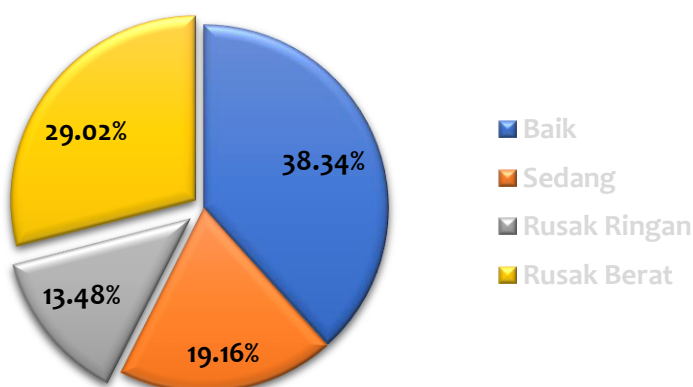
Grafik II.13 Kondisi Jaringan Jalan Provinsi Sulawesi Selatan Tahun 2018
